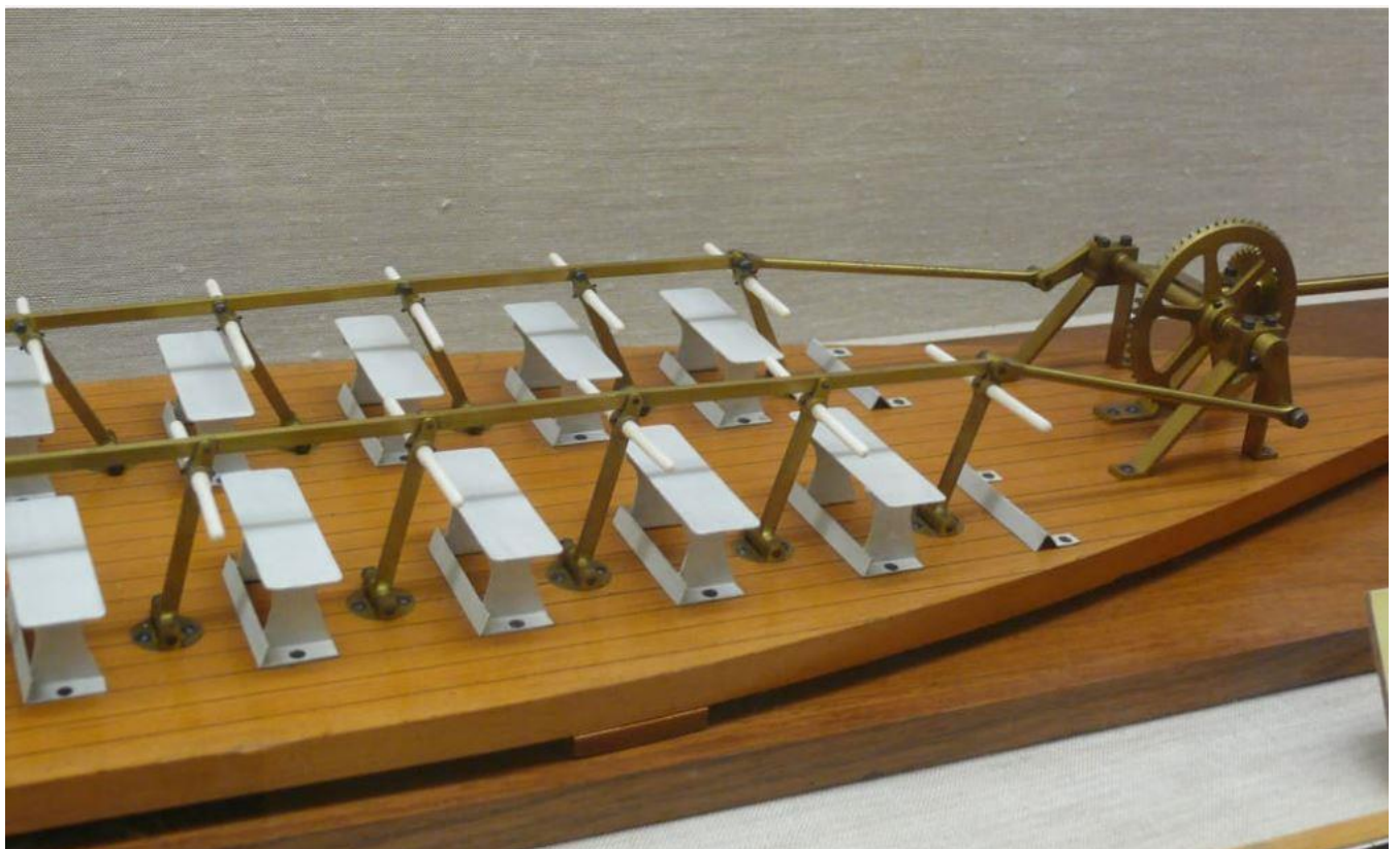
Sköld maskineri modell SSHM
