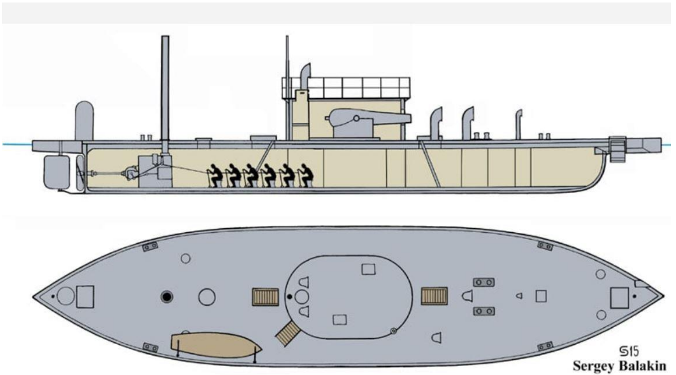
Схема установки ручного движителя монитора «Скьольд»
